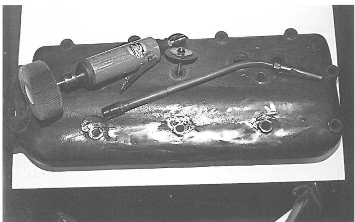
Færdigt arbejde. Luftsliber med smergelrundel og den slidte skæreskive. Svejsesbrænderen er den største i brændersættet.
