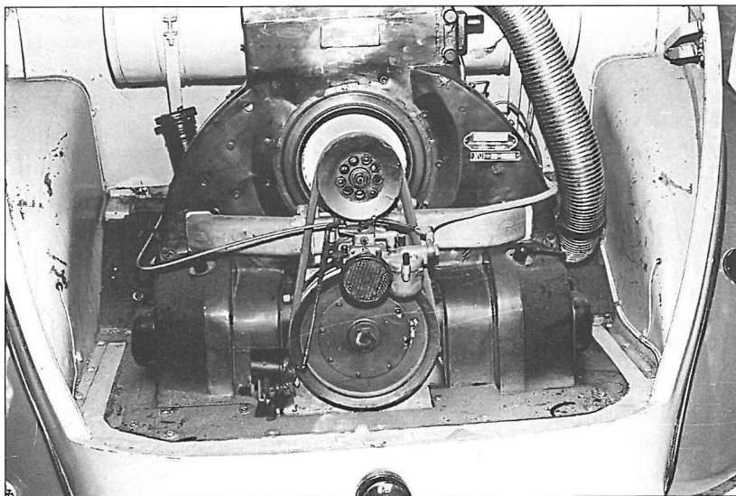
Boxermotor anno 1934.
