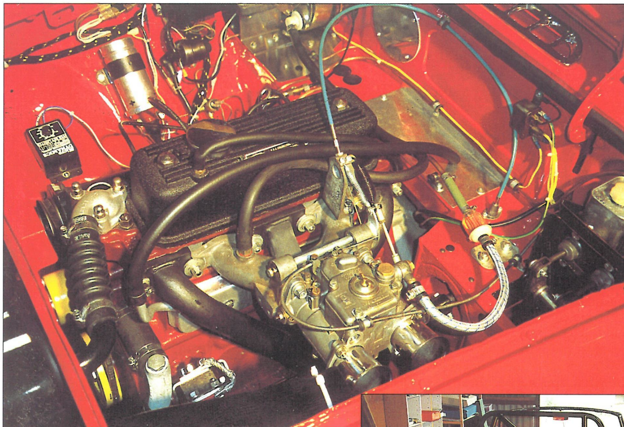
1845 ccm, M.G. A twin cam plejlstænger, smedede stemp- ler, alle bevægelige dele vægtjusteret og afbalanceret, effekt ca. 125 hk
