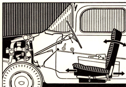
Forsædet kan indstilles under kørslen; de todeltede ryglæns hældningsvinkel kan ligeledes indstilles separat under kørslen.
