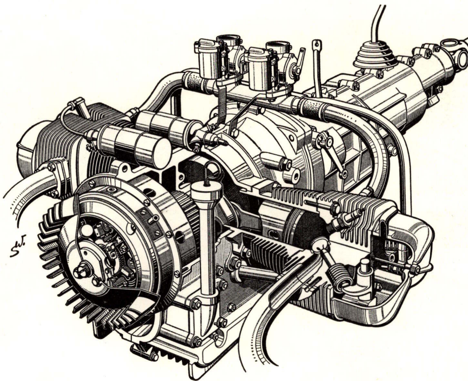
Den Store Goggomobils mekanisk fuldendte firetakts boxermotor fås i Danmark med 700 cm 3 og 30 hk. Cirkulations-tryksmøringen sker ved oliepumpe, luftkølingen ved en blæser anbragt på den forreste ende af krumtapakslen, hvorved smøring og køling reguleres automatisk i forhold til det øjeblikkelige motor-omdrejningstal.
