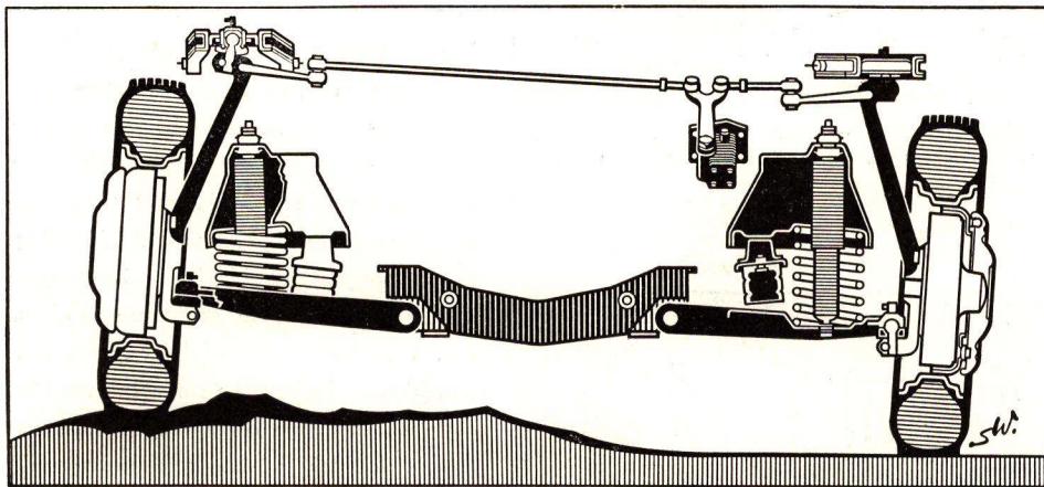
Forhjulene er uafhængigt affjedrede med skruefjedre og progressivt virkende gummifjedre. Dobbeltvirkende hydrauliske støddæmpere og snekestyring giver stor kørselskomfort.
