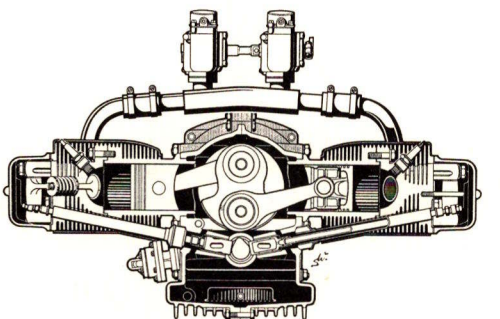
I Goggomobilen bevirker de modsatstillede cylindre i firetakts-boxermotoren en næsten fuldkommen balance. Cirkulations-tryksmøringen sker ved en oliepumpe.
