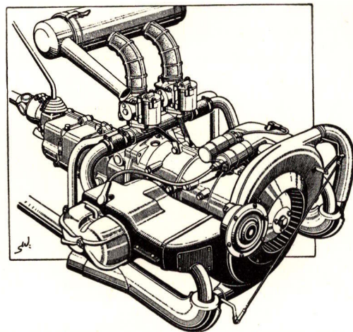
Firetakts-boxermotoren, type Glas, er forsynet med en køleluftsblæser, der er placeret foran i den naturlige luftstrøm og giver nøjagtig afpasset køling af cylindrene under alle kørselsforhold. Opvarmningsluften blæses ind i vognens indre med det nødvendige tryk, uafhængigt af kørehastigheden.
