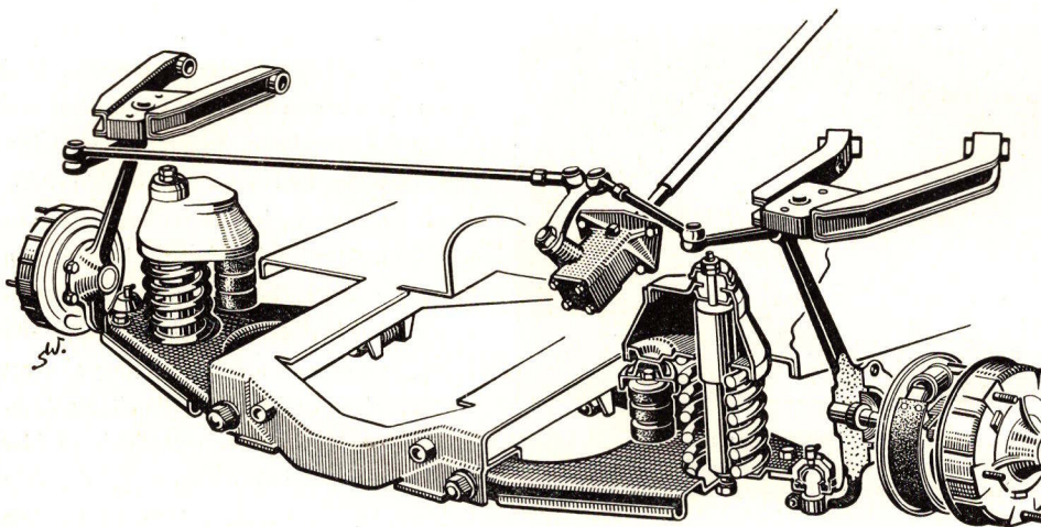
Den uafhængige affjedring opnås ved langsvingarme foroven og tværsvingarme forneden, understøttet af skruefjedre, progressivt virkende gummifjedre og dobbeltvirkende hydrauliske støddæmpere.
