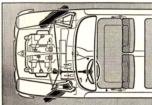
Forhjulenes gode underdrejning har muliggjort en vendediameter på kun 9 m.
