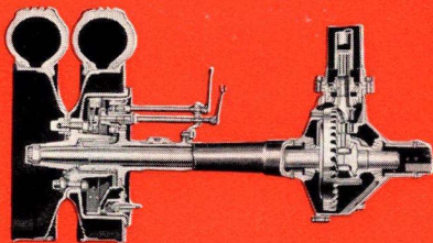
Bagaksel af \frac{3}{4} flydende Type.
