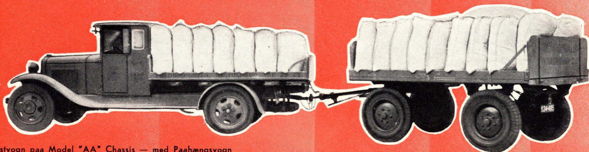
Lastvogn paa Model "AA" Chassis — med Paaheangsvogn
