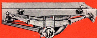
De nye halvelliptiske Bagfjedre med Hjælpefjedre.
