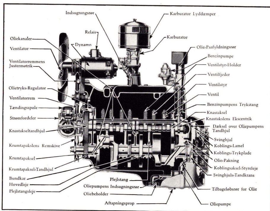
Snit af V-8 Motoren
