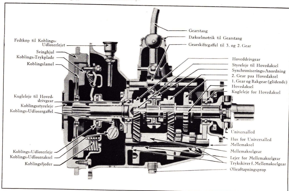
Snit af Model „Y“ og „C“ Transmissionen
