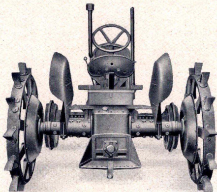
Radrenser-Traktoren indstillet til 72" Sporvidde
