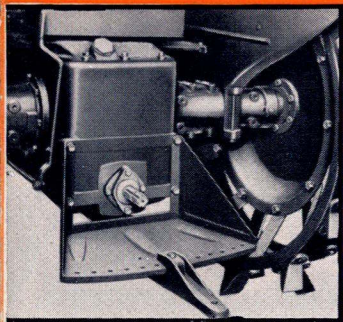
Ny Kraftoverføring, centralt anbragt. Ny, drejelig Trækbom
