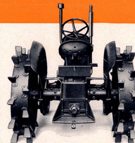
Standard-Traktoren set bagfra
