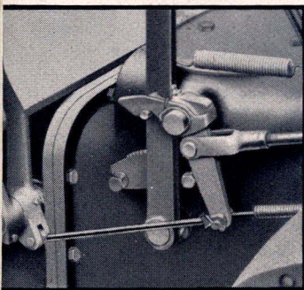
Ny Transmissions-Haandbremse
