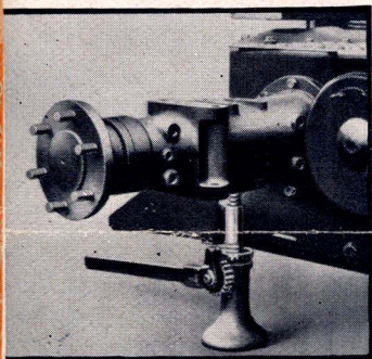
Nyt Bagakselhus med Gevindhuller til Fastgørelse af Redskaber
