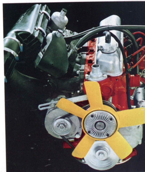
B 20 B. 2 liters, 4-cylindret. 118 hk SAE. Rensning af udstødning er standard. (Billedet viser motoren i Volvo 140-serien.)
