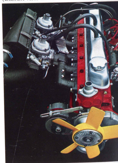
B 30. 3 liters, 6-cylindret. 145 hk SAE. Rensning af udstødning er standard.
