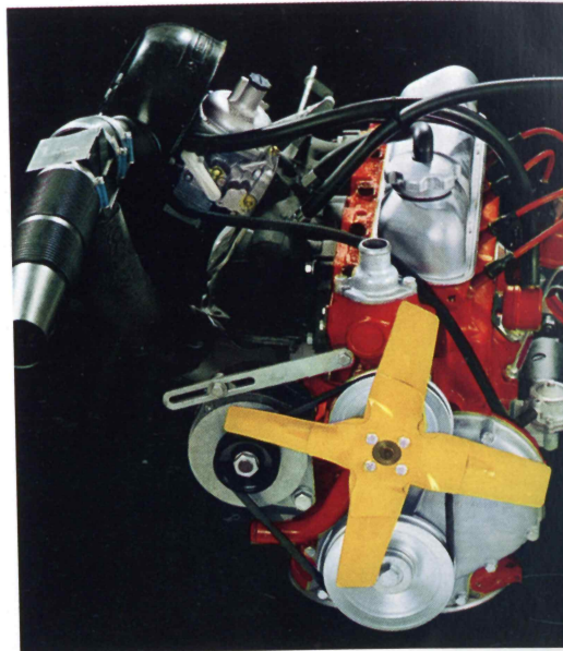
B 20 A. 2 liters, 4-cylindret. 90 hk SAE. Rensning af udstødning er standard.
