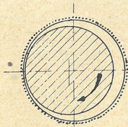
Fig 3. Her ser man, hvorledes Akslen saa at sige »klatrer« opad i Lejet under sin Rotation som Følge af det forskellige Olietryk paa Akslens Over- og Underside.
