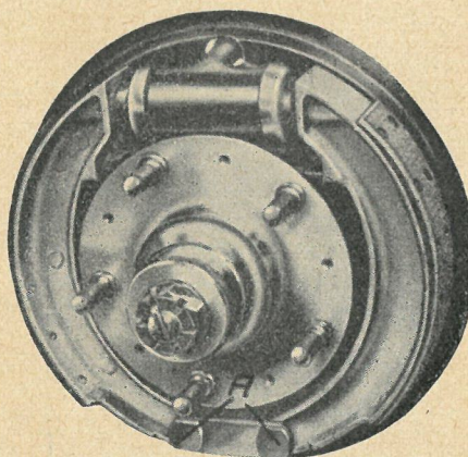
Fig. 4. Hydraulisk Bremse. De to Ankertoppe ses forned, betegnet med A.
