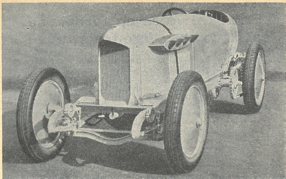
Blitzen-Benz bygget i 1909. Læg mærke til kædehjulene og de indstillelige friktionsdæmpere ved forhjulsaffjedringen.
