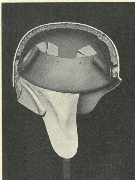
En gennemsåret hjelm af den foreslåede type. Læg mærke til den tykke foring med kork under skallen.
