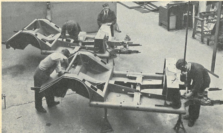
Chassiserne til Jensen 541 bliver ligesom den øvrige vogn fremstillet som håndarbejde. Den bærende konstruktion er udformet som et platformchassis med kraftige røranger.
