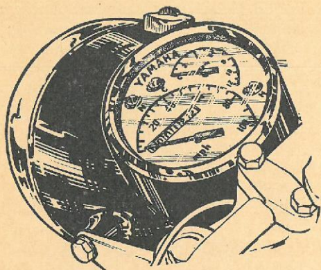
I lygtehuset er der indbygget et instrument, som indeholder såvel speedometer som omdrejningstæller, hvor det røde felt begynder ved 9000 omdr./min. Derforuden er der kontrolløys for batteriladning, frigear foroven over speedometerskalaen og nede til højre fjernlyskontrol.
