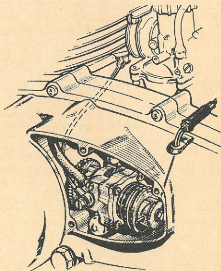
Man kommer let ind til Autolube olie-pumpen bag et dæksel på motorens venstre side. Reguleringsringen fra gashåndtaget går ned til pumpen til højre på tegningen, mens også olietilførslen til venstre cylinder er skitseret.
